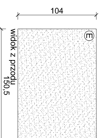
stół demonstracyjny pod dygestorium "E"
